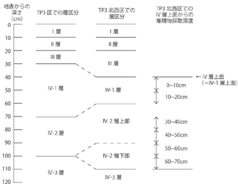
第 13 図 ツツピスキアブ洞窟の TP3 区と TP3 北西区における各層の境界の深さの対応関係、および TP3 北西区での堆積物採取深度。久貝弥嗣氏のデータによる。
