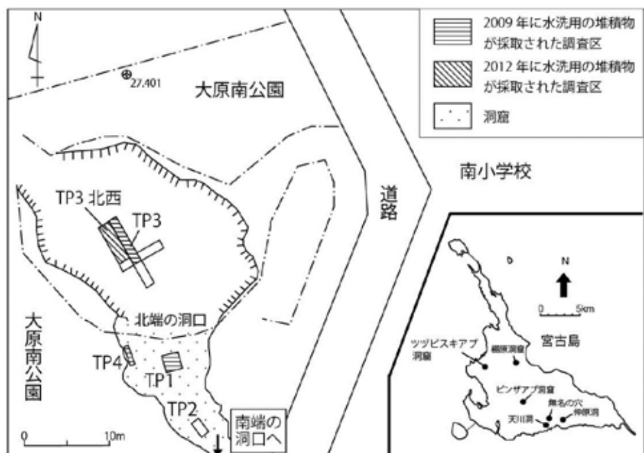
第 11 図 ツツピスキアブ洞窟の位置と発掘調査の際の調査区の配置。宮古島の代表的な第四紀哺乳類化石産地の位置も示しておいた。調査区の配置は、宮古島市教育委員会（2011）の図に加筆修正したもの。
