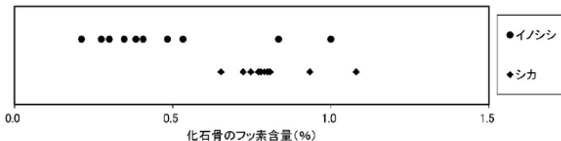
第16図. ツツピスキアブ洞窟IV－1・2層出土骨のフッ素含量
