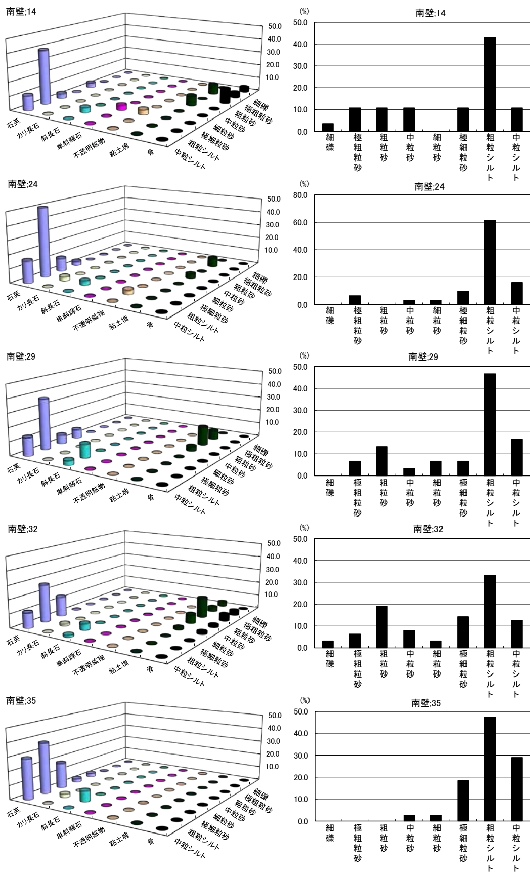
第 17 図．ツツピスキアブ洞窟における土壤中の鉱物・岩石出現頻度と粒度組成
